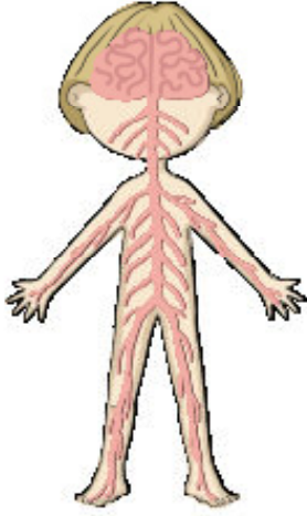
Sinir Sistemi
