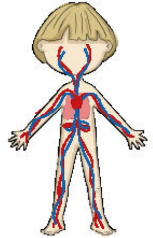
Dolaşım Sistemi
