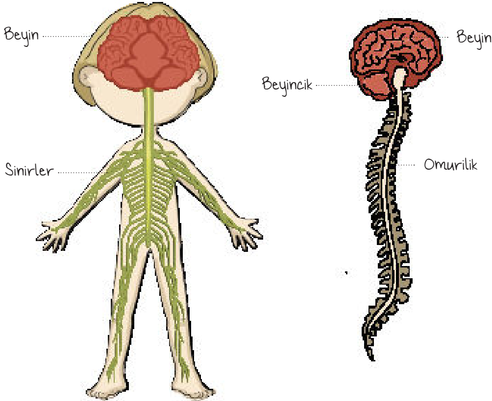
Sinir Sistemi
