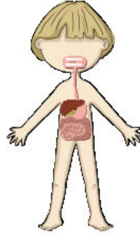
Sindirim Sistemi
