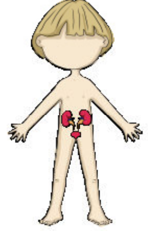
Boşaltım Sistemi
