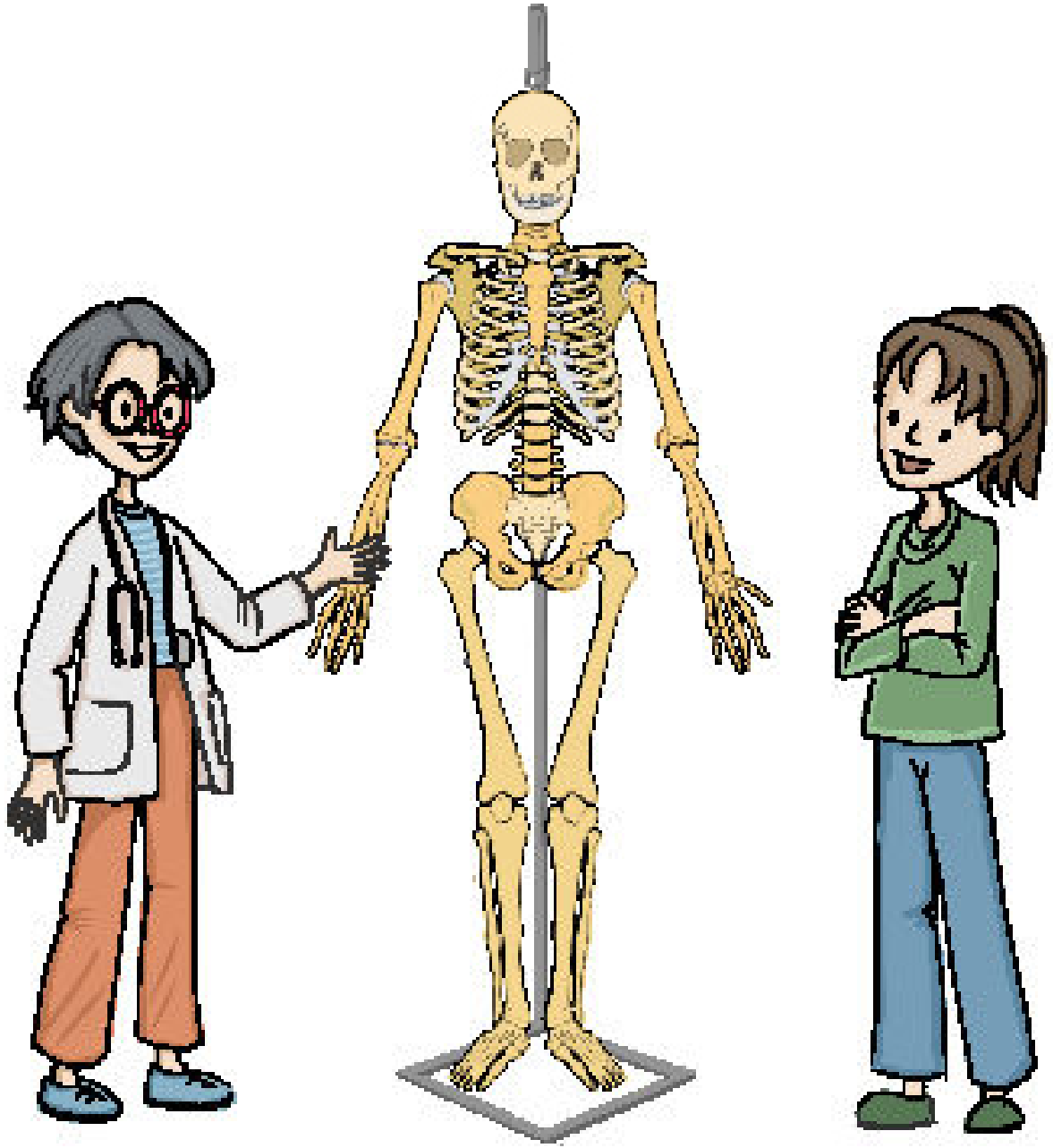
İskelet Sistemi
