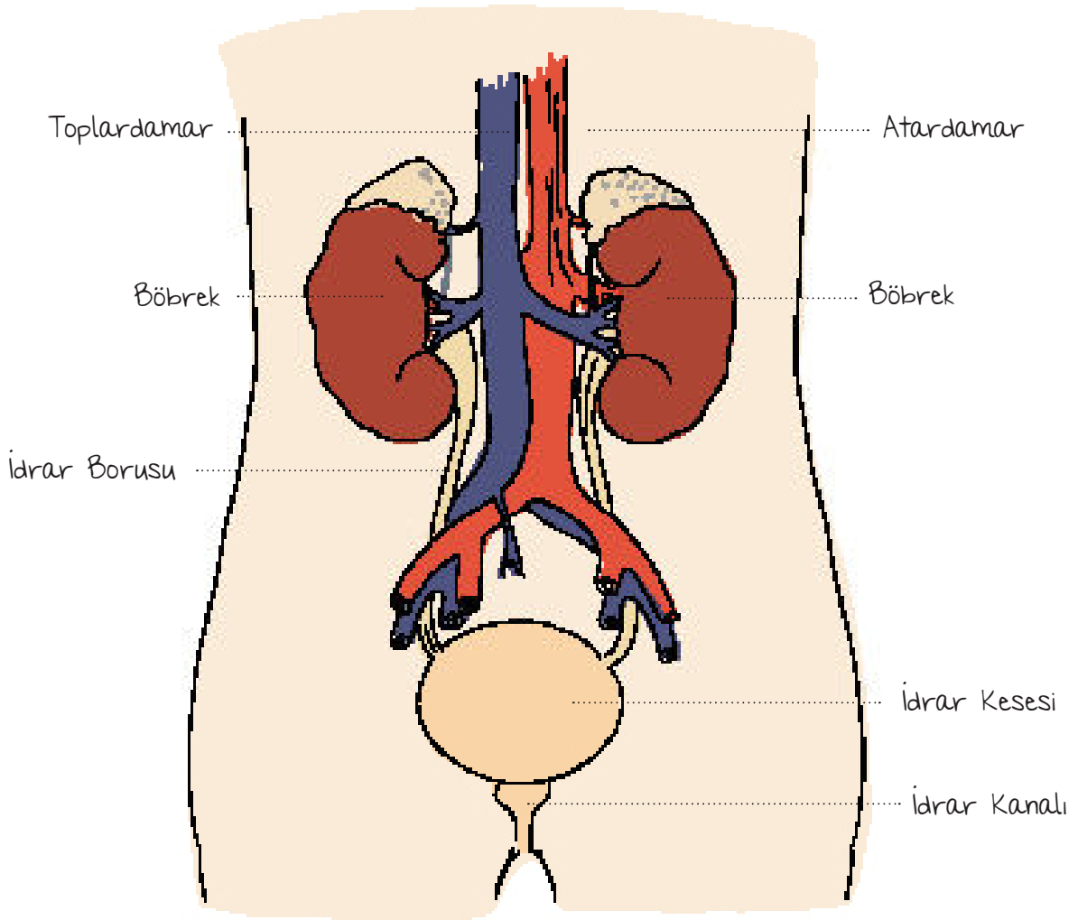
Boşaltım Sistemi
