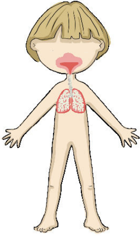
Solunum Sistemi
