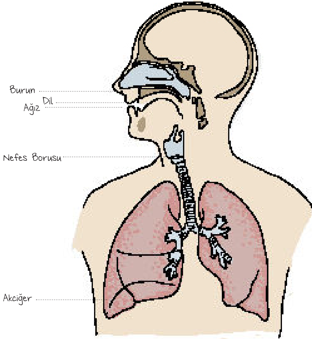
Solunum Sistemi
